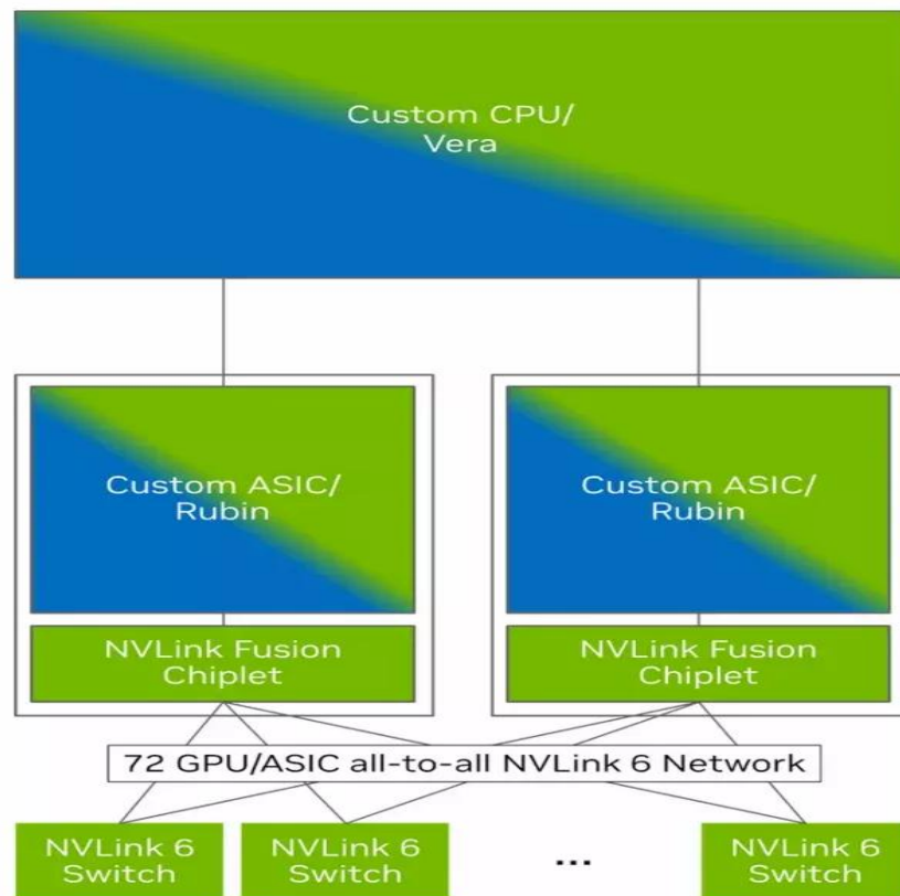
圖 6：NVLink Fusion 架構示意
