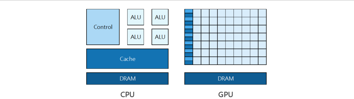
圖 11：CPU 與計算型 GPU 架構示意圖
